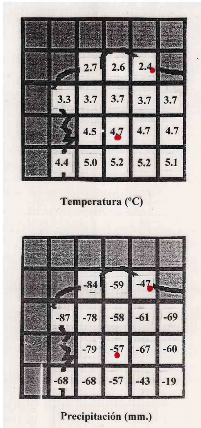
Figura 1. Predicións de cambio do modelo PRODES para Galicia nos meses de verán (xuño, xullo e agosto) para o período 2070-2100, segundo as condicións do horizonte B2. Promedios de temperatura e cantidade total de precipitación.
