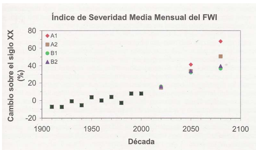
Figura 3. Evolución do Índice de Risco de Incendios para España (FWI) para o ano 2050 segundo diferentes horizontes socioeconómicos.
